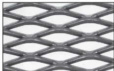
TIPO 43 - DL mm 43x10 Peso Kg/mq 10,5 sp.3 mm
