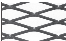
S 17 - DL mm 43x10 Peso Kg/mq 3,9 sp.1,5 mm
