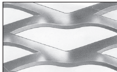
FILS 1 - DL mm 110x40 Peso Kg/mq 17 sp.4 mm
