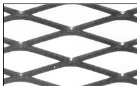
S 17 - DL 43 x 10 mm PESO kg/m 2 3,9 SPESSORE 1,5 mm
