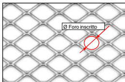
Q20 SICURA - FORO MM.10 AISI 304 PESO kg/m 2 2,4 SPESSORE 1,5 mm
