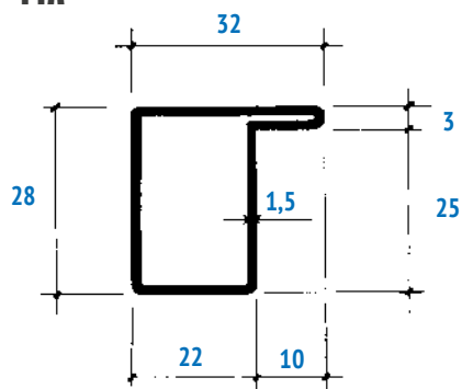
11A 1,34 kg/m (ANCHE ZINCATO)
