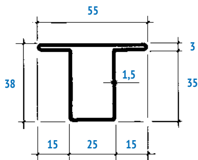
11A 1,34 kg/m (ANCHE ZINCATO)
