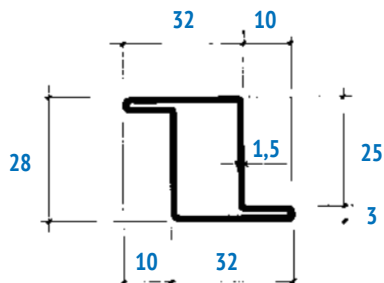
11C 1,57 kg/m (ANCHE ZINCATO)
