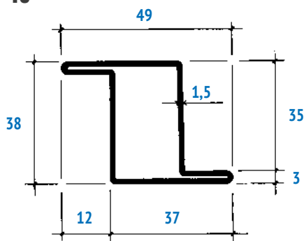
1C 1,99 kg/m (ANCHE ZINCATO)
