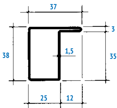
1C 1,99 kg/m (ANCHE ZINCATO)
