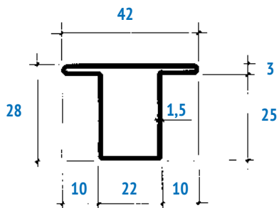
11B 1,57 kg/m (ANCHE ZINCATO)
